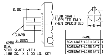
FRAME XC XE XF XD XP SC2113ATZ-LC2113ATZ 1.00 10.00 17.25 28.00 14.50 SC2512ATZ-LC2512ATZ 2.50 10.00 17.25 30.31 14.50 MC2812ATZ-LC2813ATZ 1.75 10.00 18.50 30.62 14.50
