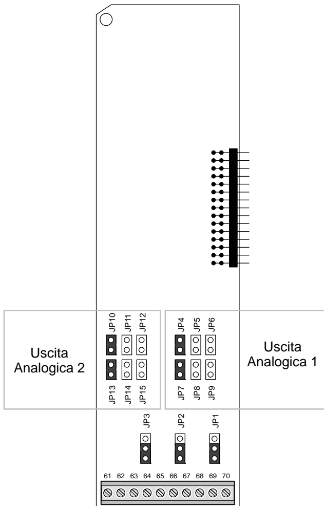
Figura 4-1 Ubicazione dei Ponticelli e Morsetti (Pianta)
